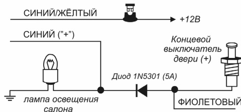
ЦЕПЬ ВНУТРИСАЛОННОГО ОСВЕЩЕНИЯ ПОЛОЖИТЕЛЬНОЙ ПОЛЯРНОСТИ
