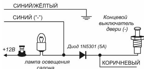
ЦЕПЬ ВНУТРИСАЛОННОГО ОСВЕЩЕНИЯ ОТРИЦАТЕЛЬНОЙ ПОЛЯРНОСТИ
